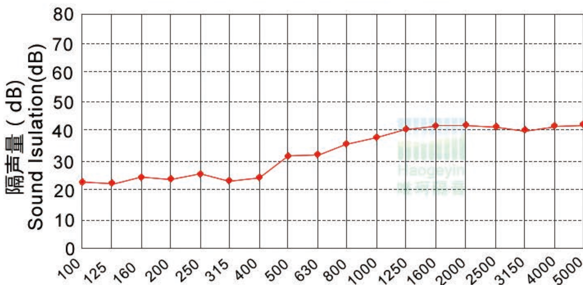
阻尼隔音板隔音数据测试图
